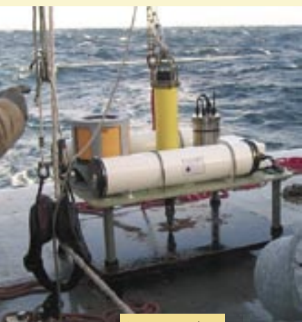
Instrumentation de détection des tsunamis.
